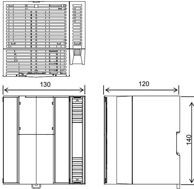
圖 1 MISR 的外形尺寸 (mm)
