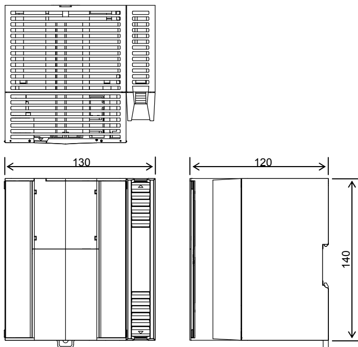
圖 1. DSS 的外形尺寸 (mm)
