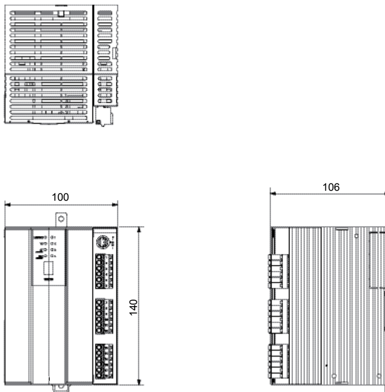
圖 1. SCS 的外形尺寸 (mm)
